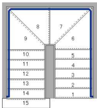
平面図
